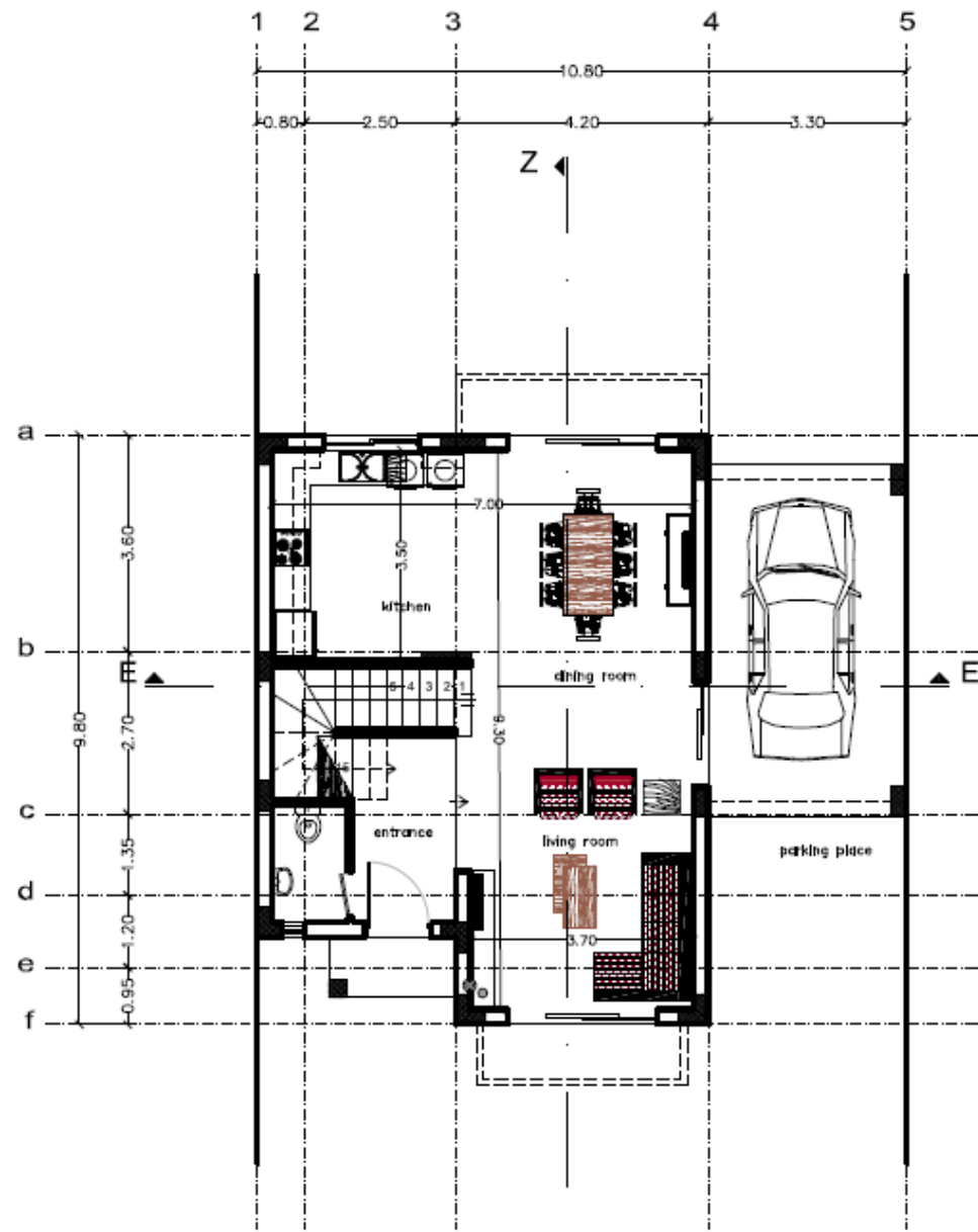
ΚΑΤΩΨΗ ΙΣΟΓΕΙΟΥ ground floor Z ←
