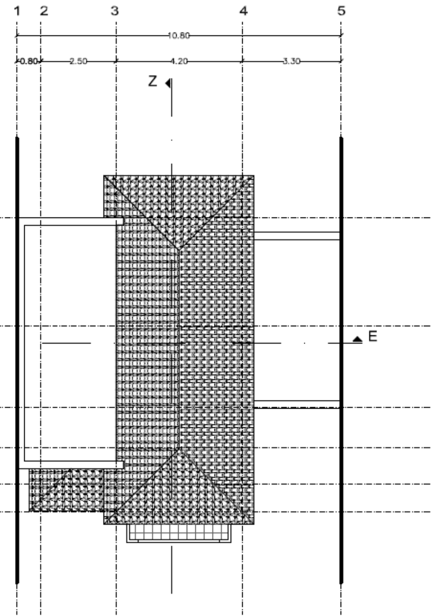
ΚΑΤΩΨΗ ΟΡΟΦΗΣ Z ←
