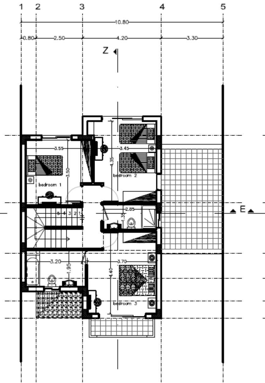
ΚΑΤΩΨΗ ΟΡΟΦΟΥ upper floor Z ←
