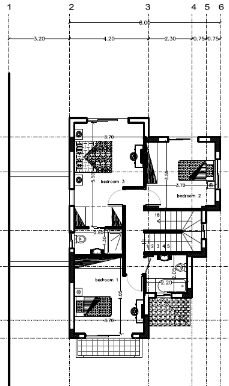
ΚΑΤΟΨΗ ΟΡΟΦΟΥ upper floor
