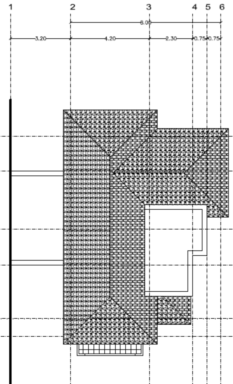
ΚΑΤΟΨΗ ΟΡΟΦΗΣ
