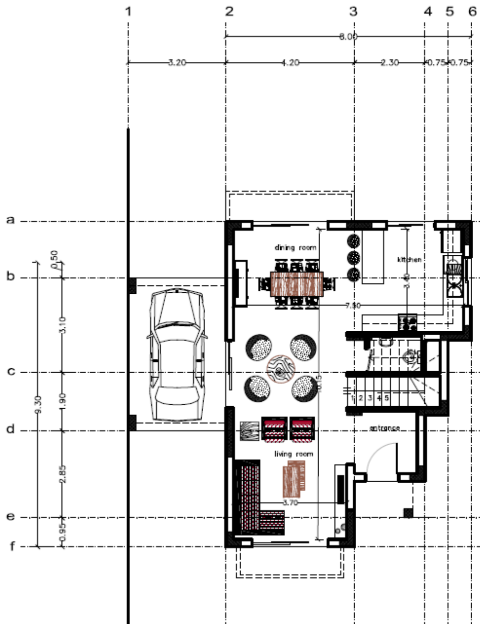
ΚΑΤΟΨΗ ΙΣΟΓΕΙΟΥ ground floor
