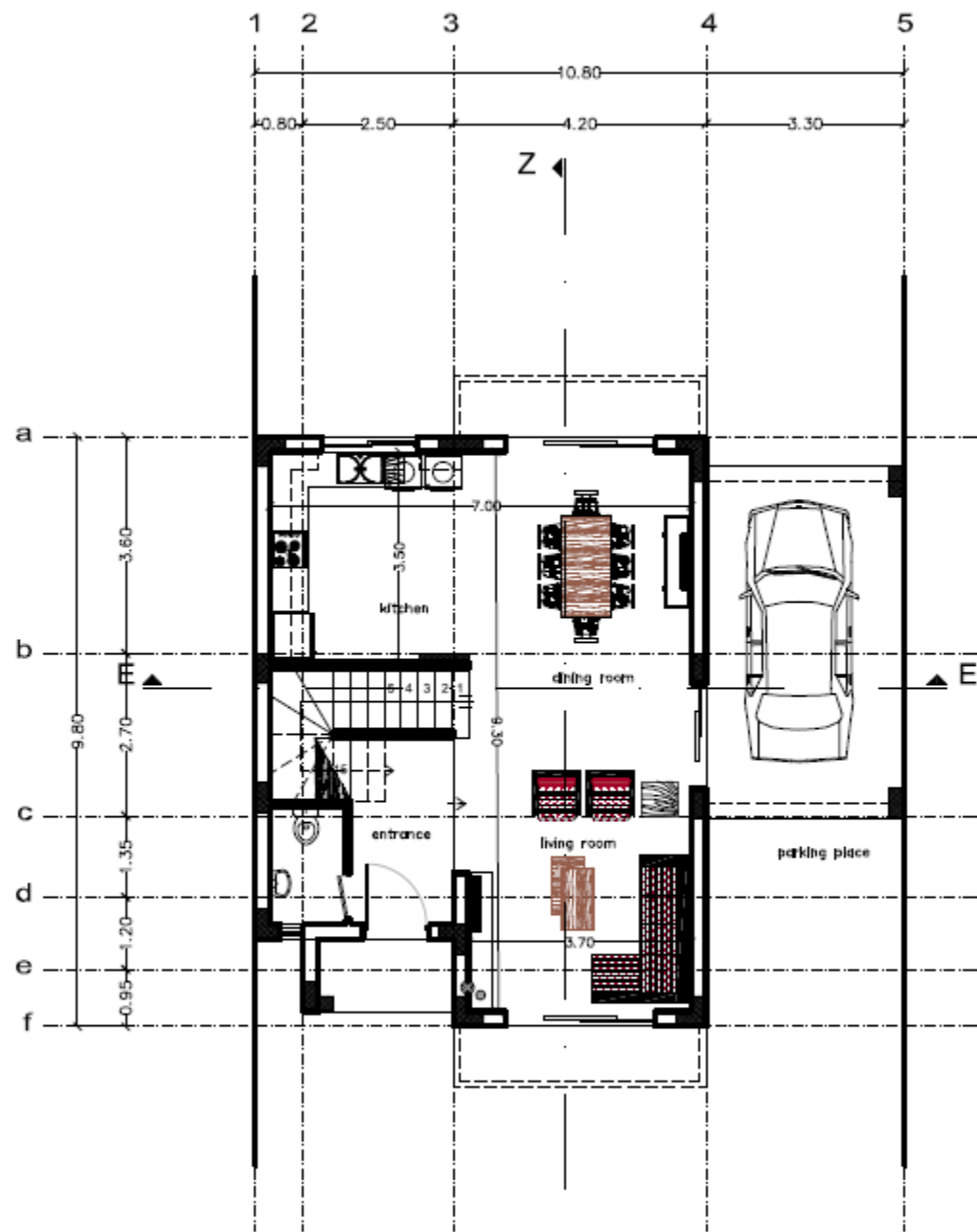
ΚΑΤΟΨΗ ΙΣΟΓΕΙΟΥ ground floor Z ←
