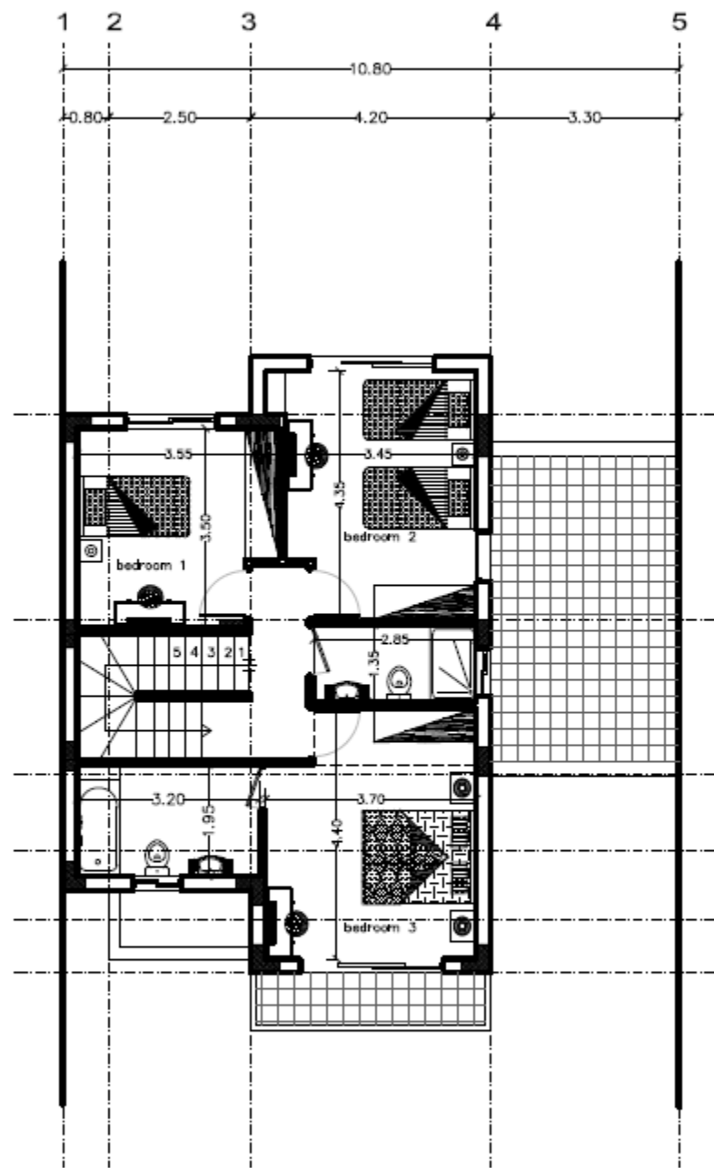
ΚΑΤΟΨΗ ΟΡΟΦΟΥ upper floor
