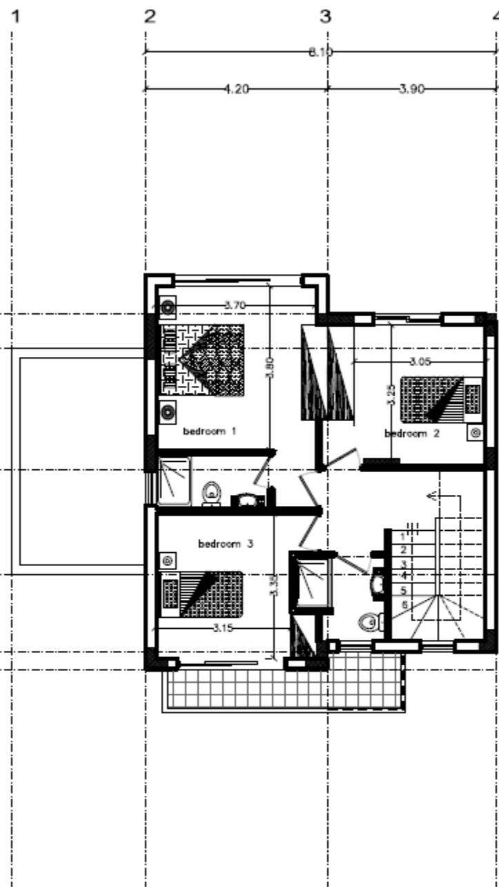
ΚΑΤΟΨΗ ΟΡΟΦΟΥ upper floor
