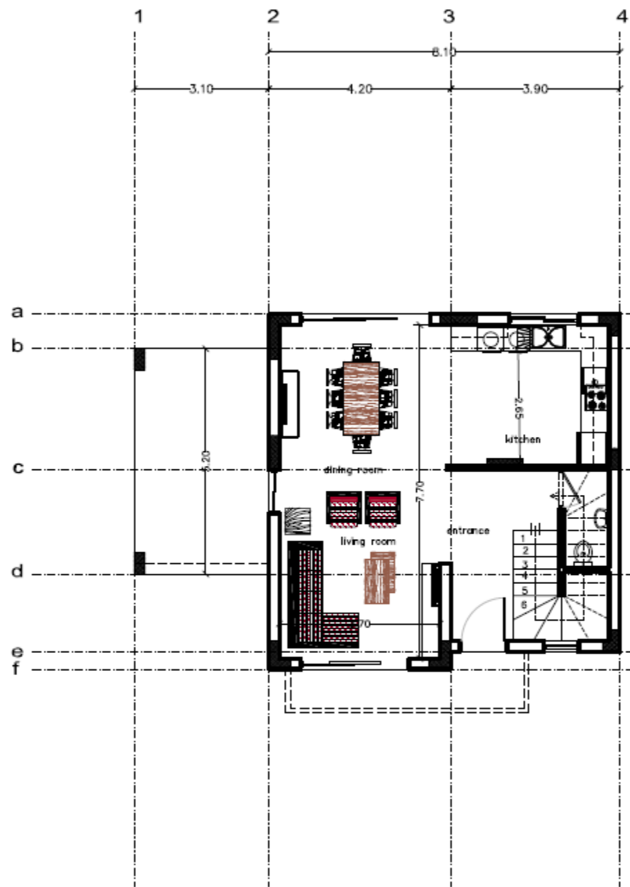
ΚΑΤΟΨΗ ΙΣΟΓΕΙΟΥ ground floor
